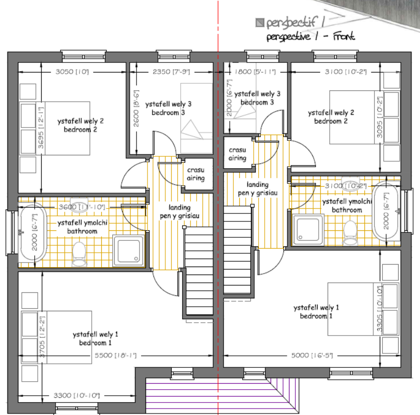
■ llawr cyntaf first floor - 1:50
